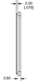
SIDE OF LID
